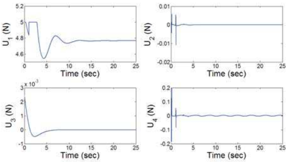
Fig. 5. Control inputs
