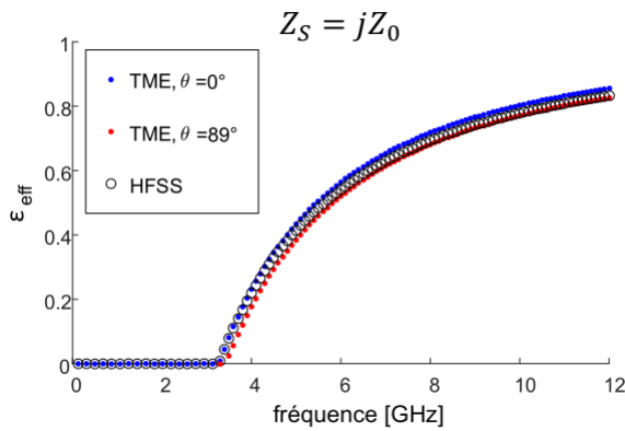
Figure 2. Courbe de dispersion sans correction en \theta
